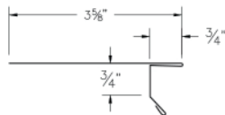
60 Drip Edge (ABSDEcc)
